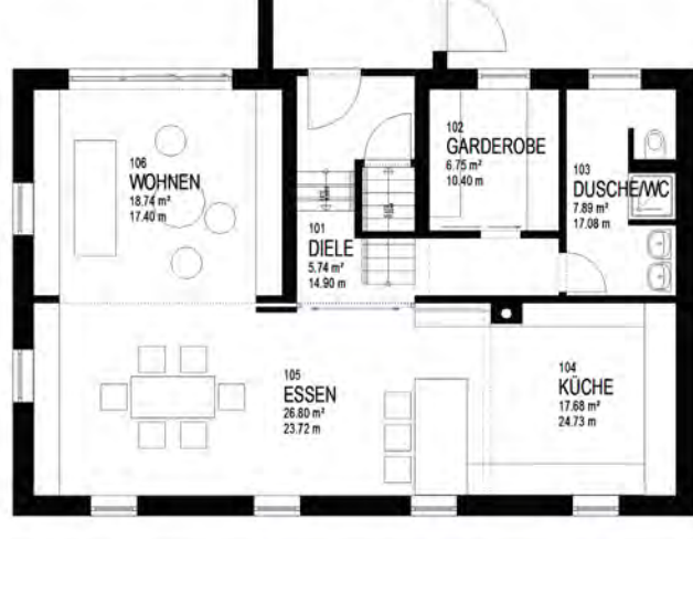
Planung Erdgeschoss
